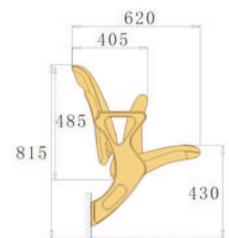
Kotvení do boku nízkého stupně
