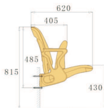
Kotvení do boku vysokého stupně
